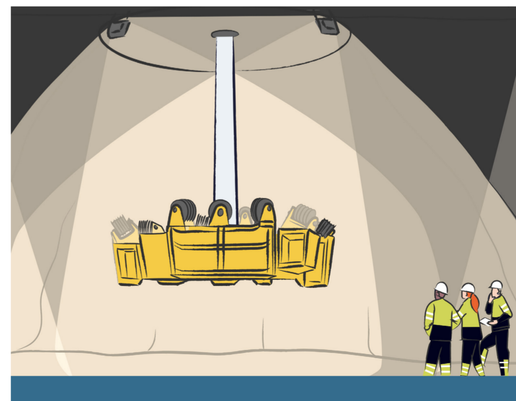
Illustration du Raise Boring, méthode de percement retenue pour réaliser les puits d'aération du tunnel de base à Avrieux. Un train de tiges équipé d'un outil de percement remonte vers la surface en enlevant la matière qui tombe par gravité. A droite, photos de la chambre de pied des puits d'Avrieux avec tige-pilote et outil.
