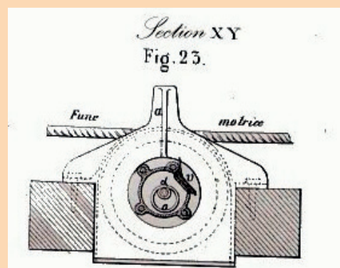
Une poulie de support, la position et la section du câble d'Agudio selon les plans de Alberto Olivetti
