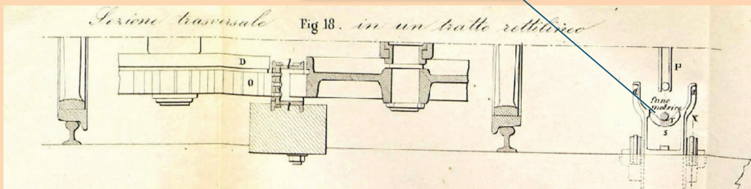
Une poulie de support, la position et la section du câble d'Agudio selon les plans de Alberto Olivetti
